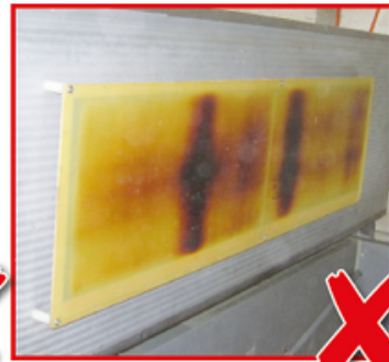
Heizelement mit Hotspot (überhitzter Bereich)
